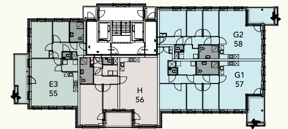
Zesde verdieping
