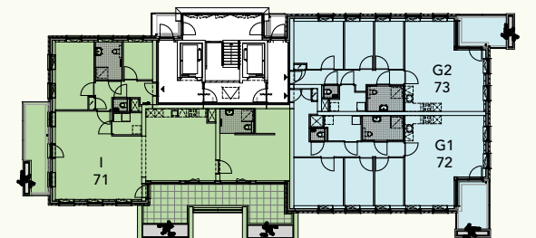
Tiende verdieping
