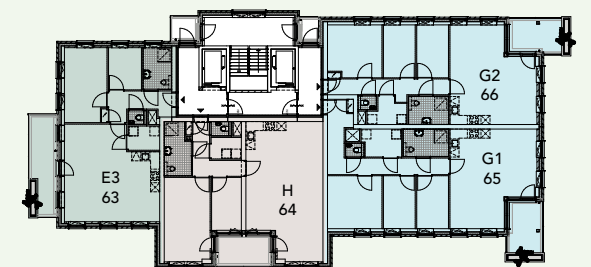
Achtste verdieping
