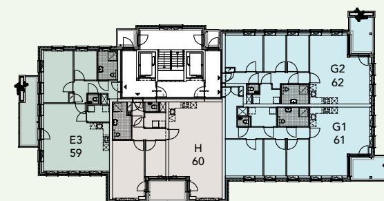
Zevende verdieping
