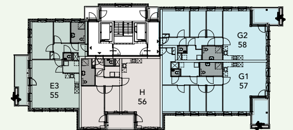
Zesde verdieping
